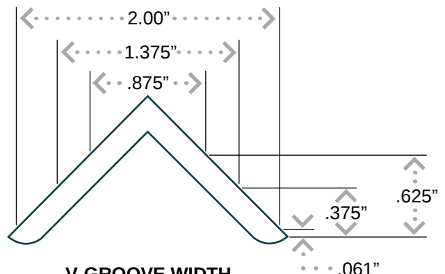
V-GROOVE WIDTH
