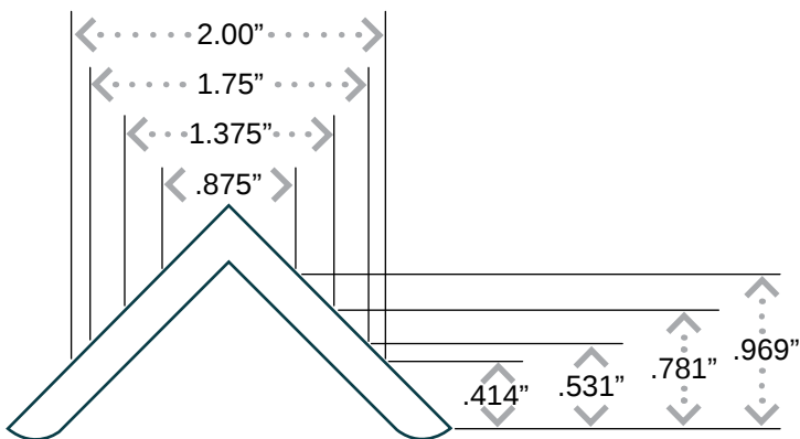
V-GROOVE WIDTH
